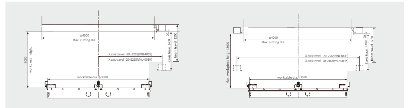
VNL400D/DK
